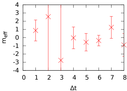
F_2: \phi^{(2)}
