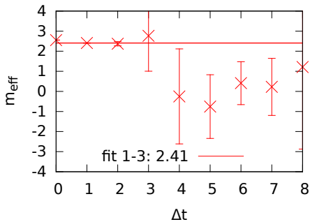
U_2: \phi^{(2)*}\phi^{(2)}
